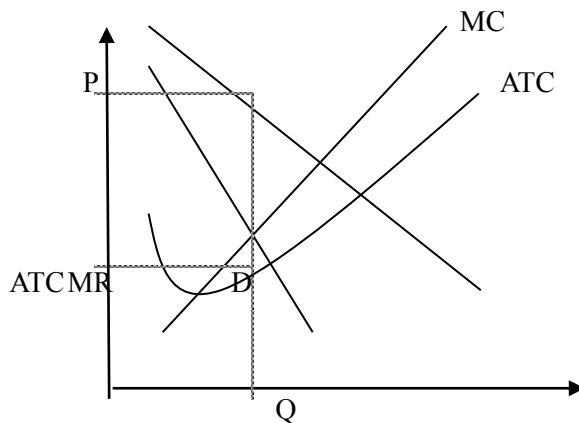
ნახ. 1. კომპანიების მოგების მიღების პირობა
