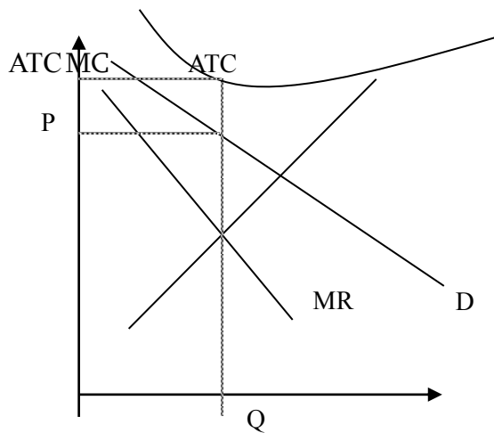
ნახ. 2. კომპანიების ზარალის მიღების პირობა
