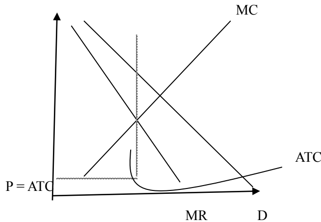
ნახ. 3. მოგება გრძელვადიან პერიოდში
